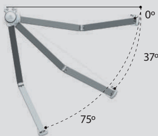
Τοίχου
